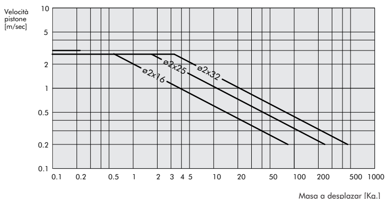
Grafico de amortiguacion
